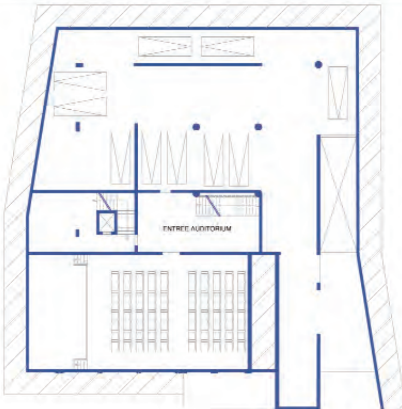
PARKING- AUDITORIUM- PLAN SOUS-SOL2- (N.T.S)
